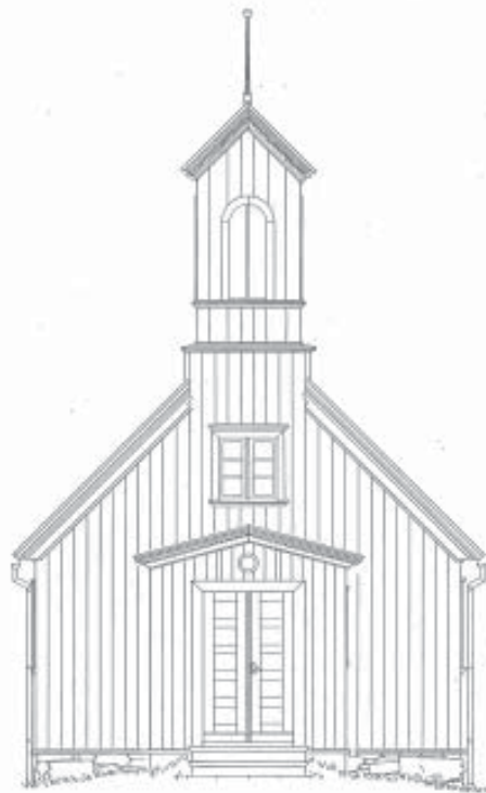
Reynistaðarkirkja (1868-1870) uppmælingauppráttur eftir Jón Pálsson
