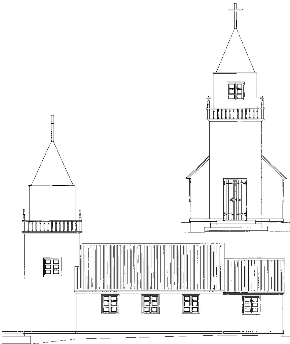
7. Framstafn og suðurhlið í mkv. 1:100. Mælt og teiknað Per Kruse og Mogens Brandt Poulsen arkitektar. – Front and south elevations to a scale of 1:100. Survey and plans by architects Per Kruse and Mogens Brandt Poulsen.
