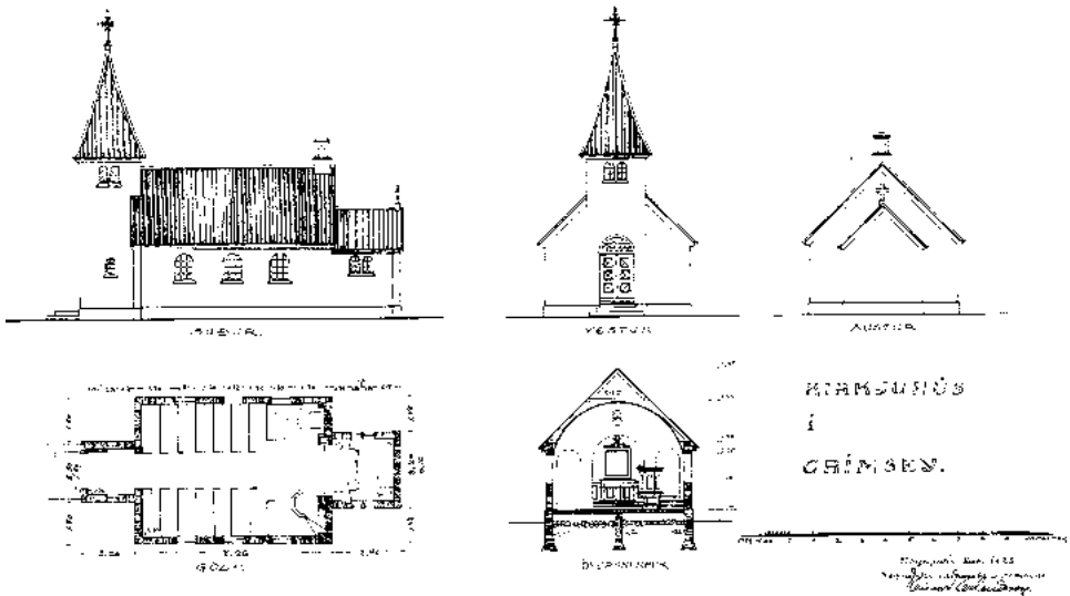
4. Tillaga Guðjóns Samúelssonar húsameistara ríkisins að steinsteyptri kirkju í Grímsey dagsett í desember 1925. Teikning gerð í mkv. 1:100 en sýnd hér í mkv. 1:350. – Design for a concrete church on Grímsey island by State Architect Guðjón Samúelsson, dated December 1925. Plan to a scale of 1:100, shown here 1:350.
