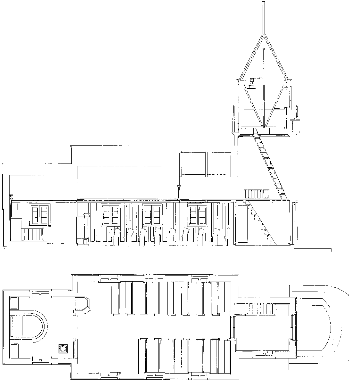
6. Grunnmynd Miðgarðakirkju og langskurður í mkv. 1:100. Mælt og teiknað Per Kruse og Mogens Brandt Poulsen arkitektar. – Plan and longitudinal section of Miðgarðar Church to a scale of 1:100. Survey and plans by architects Per Kruse and Mogens Brandt Poulsen.
