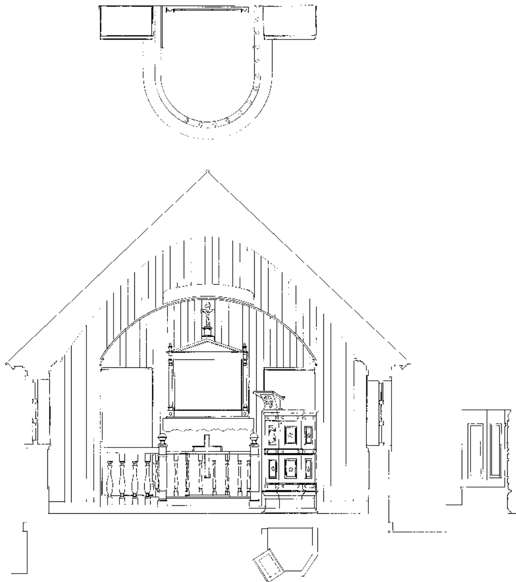
8. Þverskurður í mkv. 1:50. Mælt og teiknað Per Kruse og Mogens Brandt Poulsen arkitektar. – Cross-section to a scale of 1:50. Survey and plans by architects Per Kruse and Mogens Brandt Poulsen.
