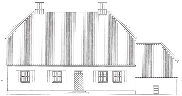
Nesstofa á Seltjarnarnesi (1763). ÞG 1979
