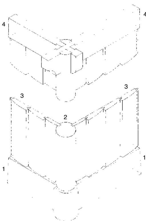
11. Stafverk. 1. aurstokkur. 2. hornstafur. 3. plægðar, standandi þiljur. 4. sylla.
