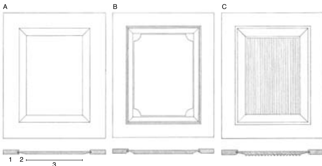
10. Spjaldapíll. A. einföld gerð spjaldapílls. 1. rammi. 2. fleygskurður. 3. háflötur. B. spjald með barokksneiddum háfleti. C. spjald með rákuðum háfleti.
