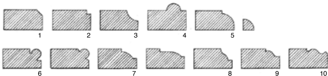
4. Hefilstrík, hefðbundin fyrri tíðar strík. 1. sneiðing, fas. 2. falsstrik. 3. húlkáll. 4. hálfstafstrik. 5. kvartstafstrik. 6. treikvartstafstrik. 7. flatstafstrik. 8. reistur karnis. 9. liggjandi karnis. 10. liggjandi karnis með sneiddri brún.
