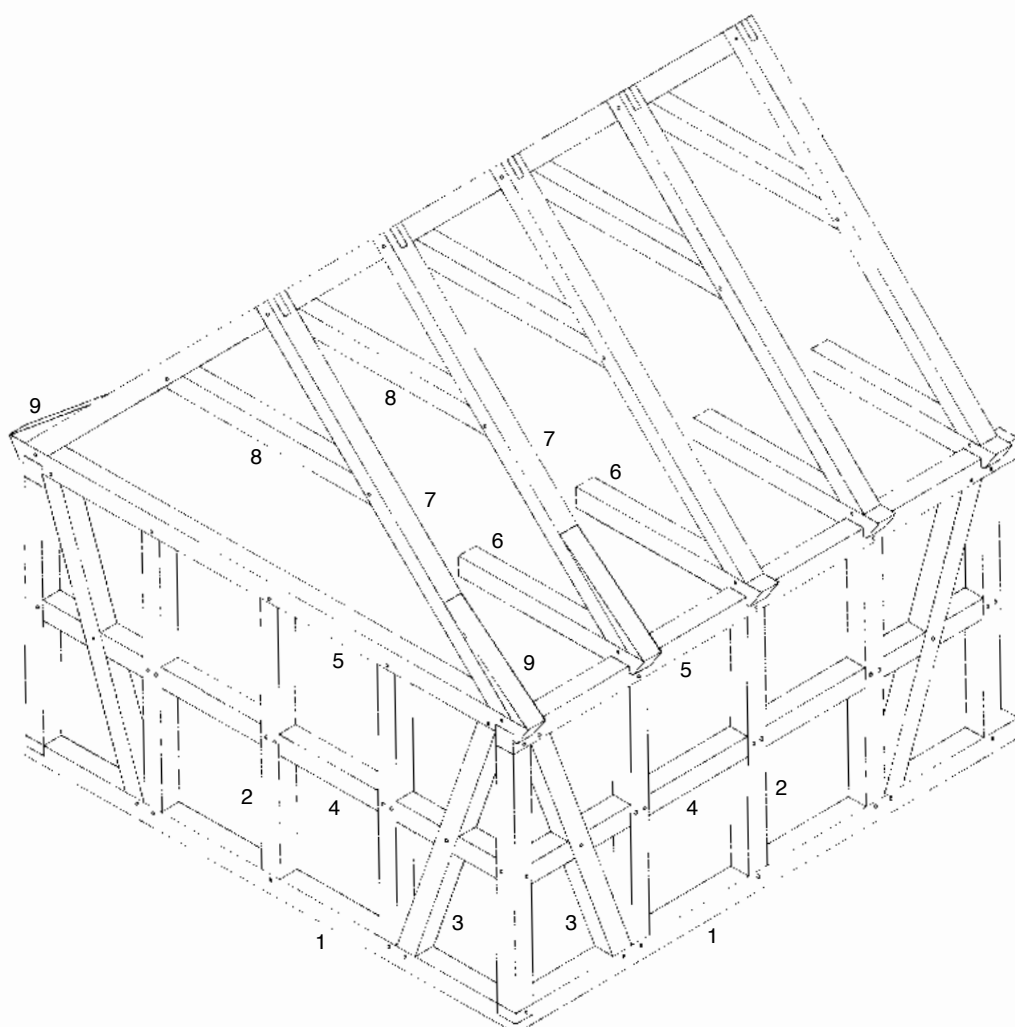
2. Bindingsverk. 1. aurstokkur, fótstykki. 2. stafur, stólpi. 3. skástífa, skakkslám, skástytta, stormband, sniðband. 4. miðsylla, skammtré. 5. sylla, lausholt, stokksylla, veggasylla. 6. bití. 7. sperra. 8. skambbiti, hanabjálki. 9. ufsasperra.
