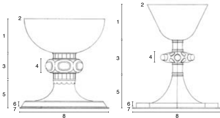
5. Kaleikar. A. rómanskur kaleikur. B. gotneskur kaleikur. 1. skál. 2. brún. 3. leggur. 4. hnúður. 5. fótur. 6. brún. 7. kantur, standkantur. 8. botn.
