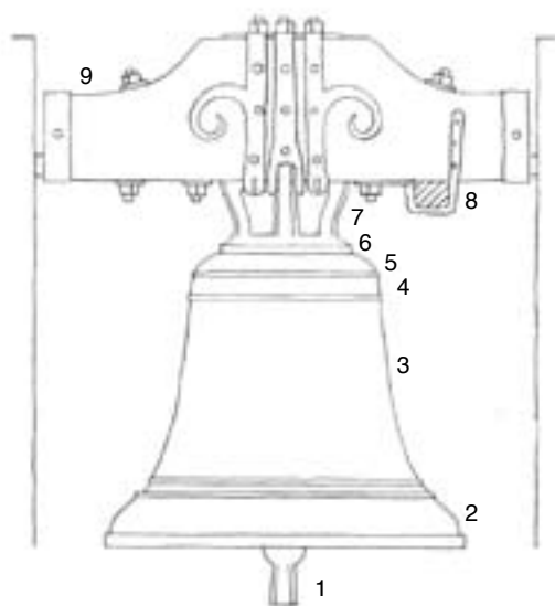
6. Kirkjuklukka. 1. kölfur. 2. slaghringur. 3. klukka. 4. háls. 5. kollur. 6. krónustétt. 7. lykkja. 8. dragstong. 9. rambald.
