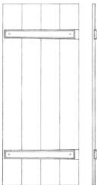
8. Okahurð. Okarnir eru litillega fleyglaga og grópaðir í plankana sem mynda hurðarflöguna.
